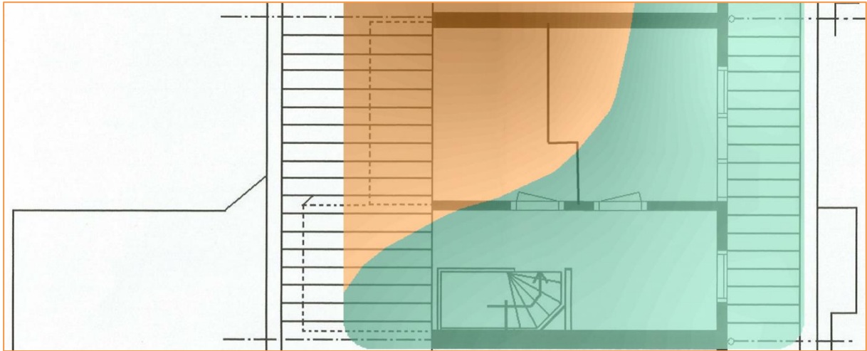
Figuur 6: Heatmap 2.4 GHz - Tweede verdieping
