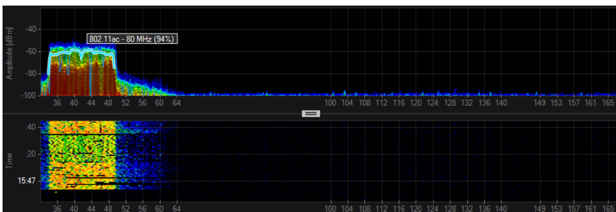
Afbeelding 6 : 5 GHz – 80 MHz
